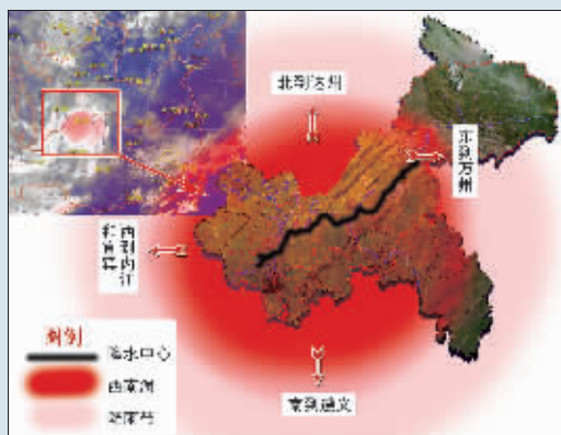
中西部被强降水带笼罩 郭娟 制图
